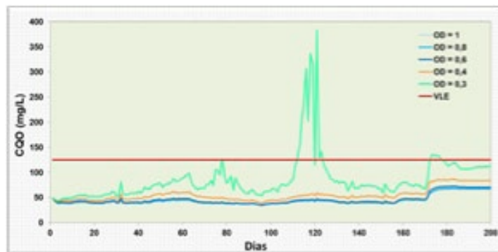
Valores simulados da qualidade do efluente final (CQO) para vários set points de oxigénio dissolvido (OD) no tratamento biológico
